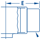
Optional 1/2" Conduit Boss
